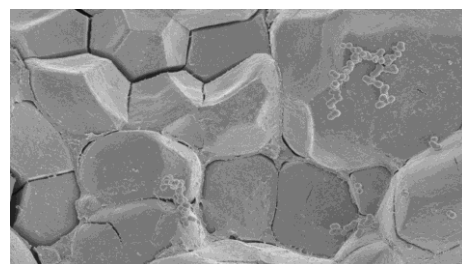
Grânulos de amido: amilose e amilopectina são os polímeros que os constituem.
